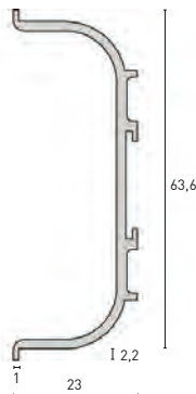
Griffmulde C-Profil horizontal
