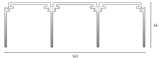
Deckenschiene dreiläufig
