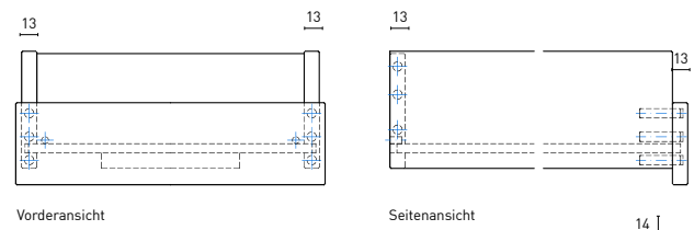
Vorderansicht
