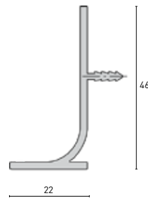
Griffmulde L-Profil vertikal
