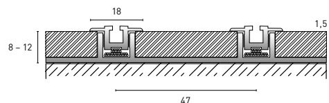
Dreiläufig zum Auflegen mit hohem Mittelsteg
