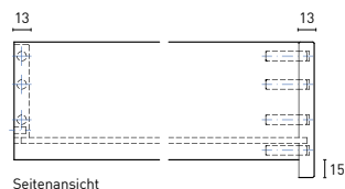
Seitenansicht
