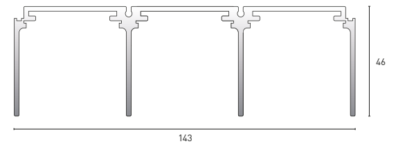
Deckenschiene dreiläufig
