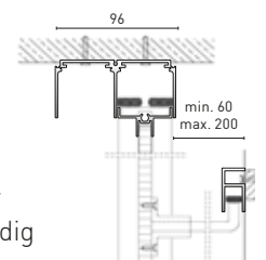
Führungsprofil für hintere Führung
