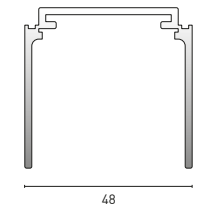
Deckenschiene einläufig
